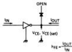
2. V_{CE(sat)} , h_{FE}
